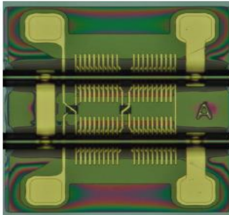
素子拡大図
